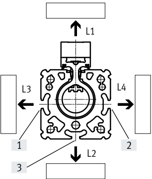
Piston Ø 18/25
